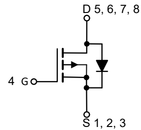
PDFN5060
